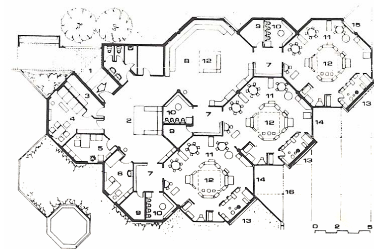
Σχήμα 4. Οργάνωση του Συγκροτήματος
