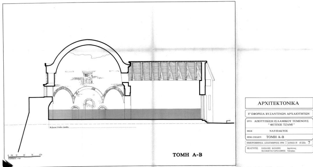
Εικ.28: Αρχιτεκτονική τομή, Φετιχιέ τζαμί
