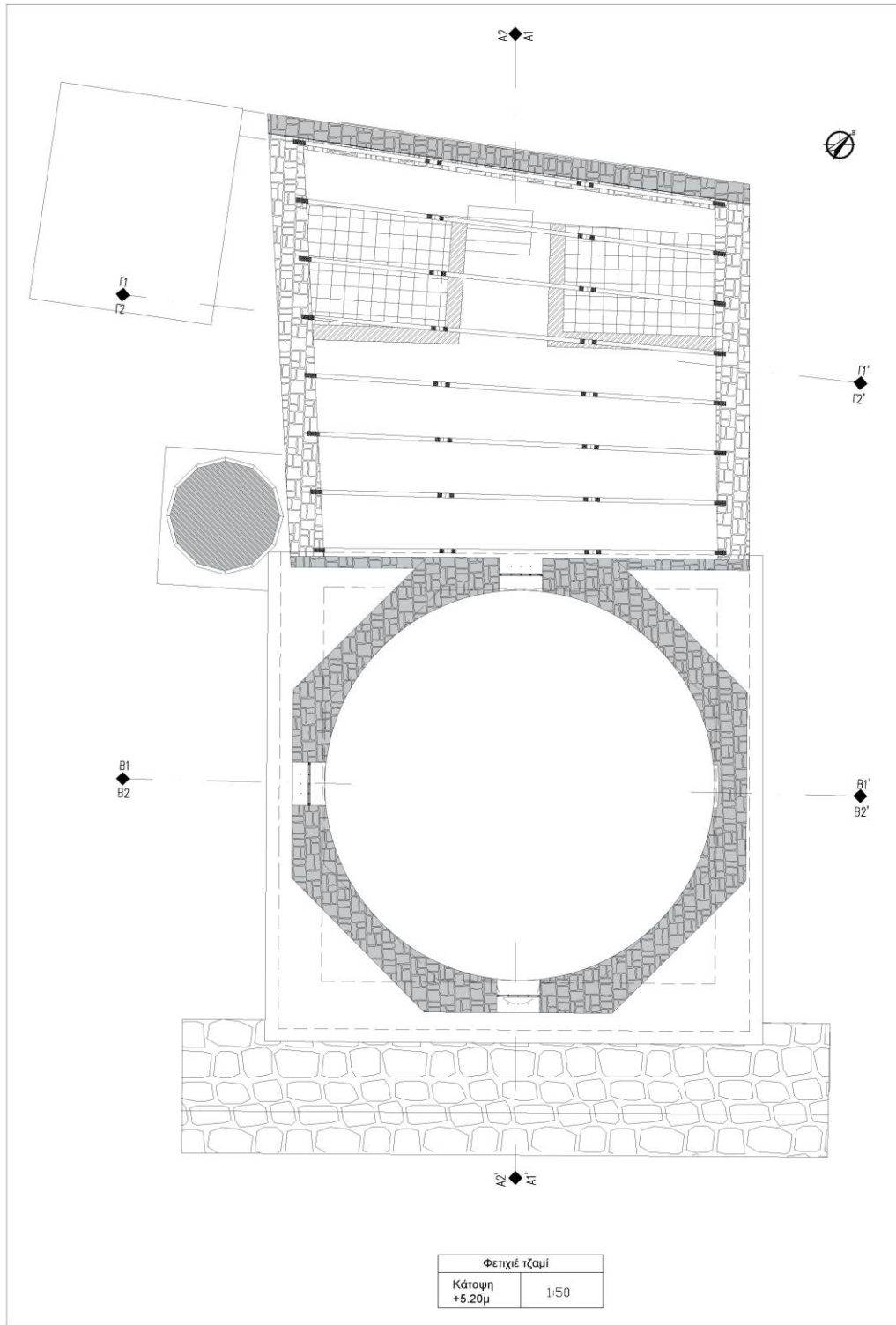
Εικ. 31 Κάτοψη +5,20μ, Φετιχέ τζαμί
