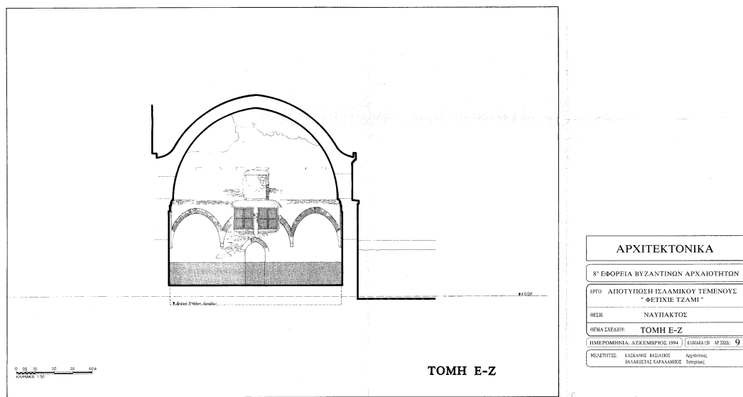
Εικ.20: Αρχιτεκτονική τομή νότιου προσανατολισμού, Φετιχιέ τζαμί
