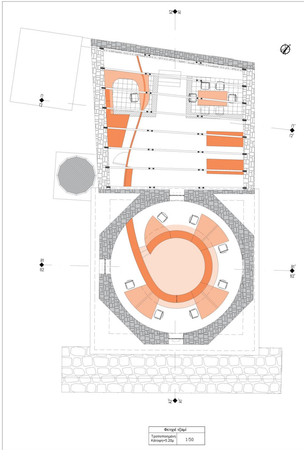
Εικ. 46 Τροποποιημένη κάτοψη +5,20μ Φετιχέ τζαμί
