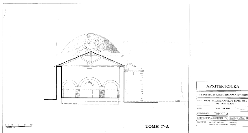
Εικ.25: Αρχιτεκτονική τομή, Φετιχιέ τζαμί (Πηγή: Χορήγηση κ. Κασκάνη)
