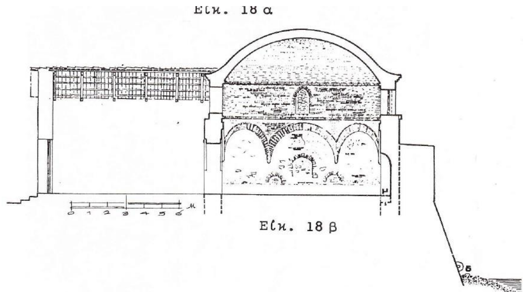
Εικ. 27 Αρχιτεκτονική τομή, Φετιγιέ τζαμί
