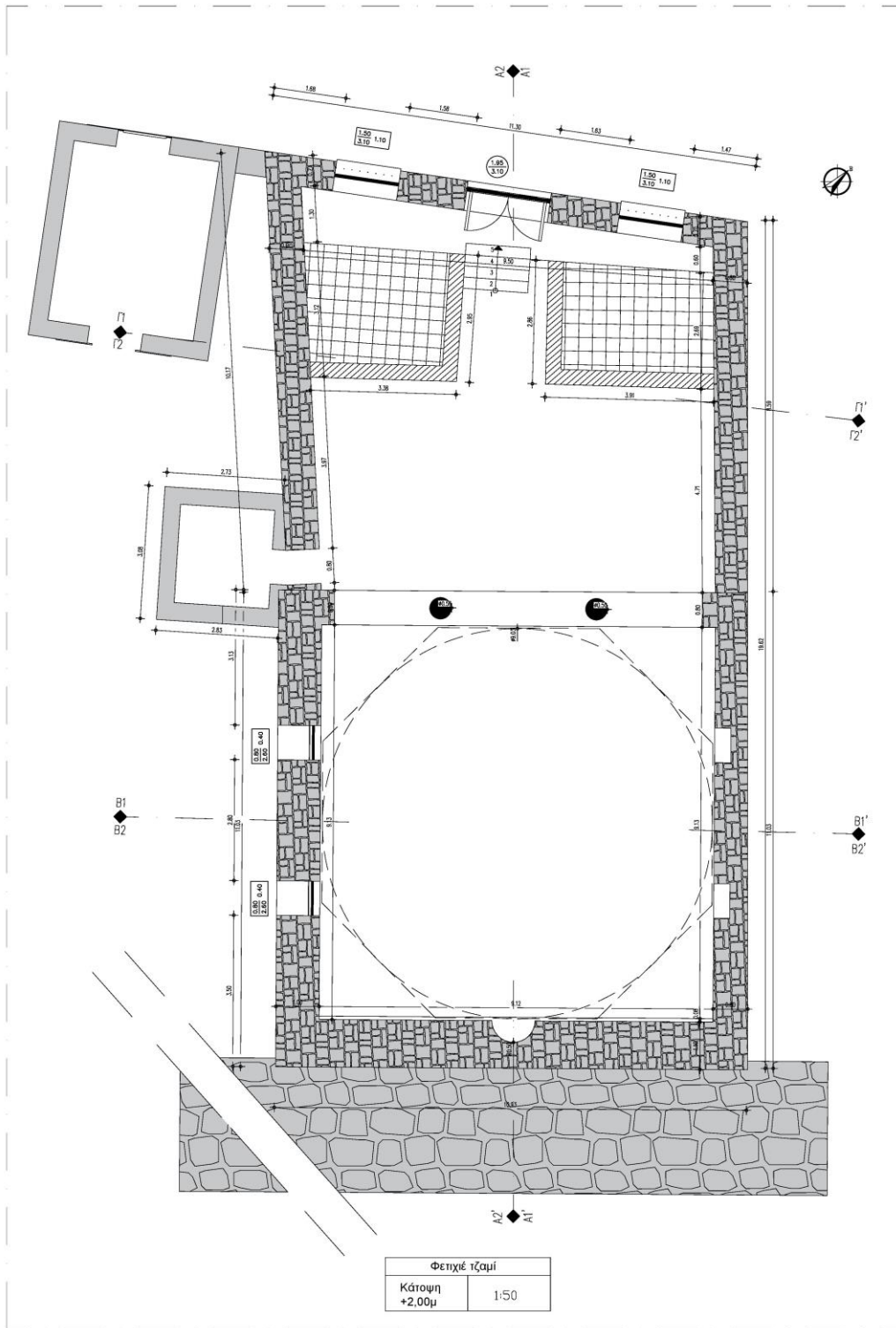
Εικ.30 Κάτοψη +2.00μ Φετιγιέ τζαμί
