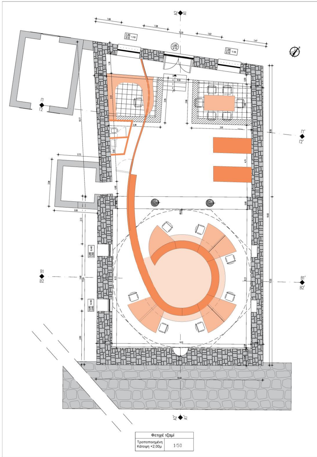
Εικ. 45 Τροποποιημένη κάτοψη +2,00μ Φετιχέ τζαμί
