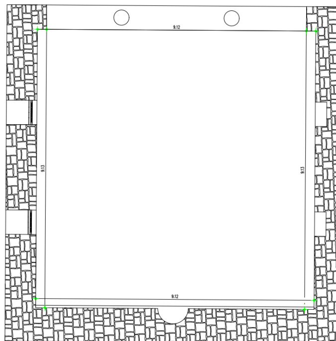
Εικ. 1: Κάτοψη Τετραγωνικής Βάσης, Φετιχιέ Τζαμί
