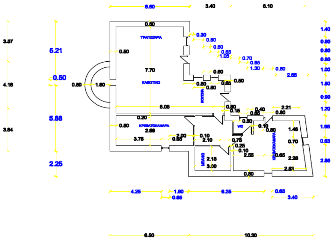
ΣΧΗΜΑ 5. Η κάτοψη της πρότασης ανακαίνισης του κτιρίου με τις ακριβώς ίδιες εξωτερικές διαστάσεις και την αναδιαμόρφωση του εσωτερικού χώρου.
