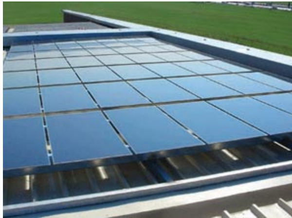
Εικ 4.9 Ενσωμάτωση άμορφων Φ/Β στο Τεχνολογικό Μουσείο Θεσσαλονίκης
