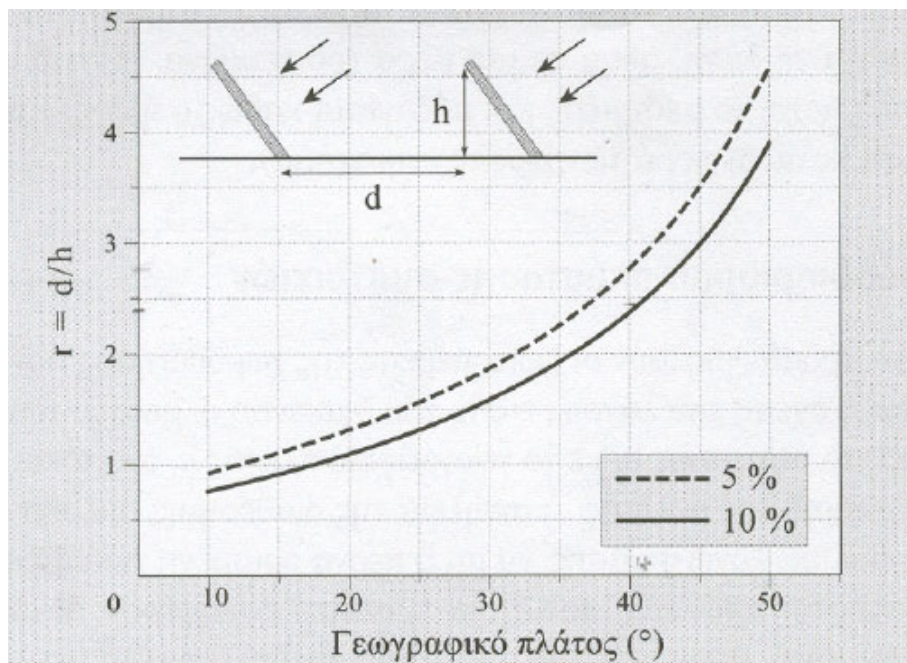
Σχήμα 2.1 Συσχετισμός του d/h συναρτήσει του Γεωγραφικού Πλάτους
