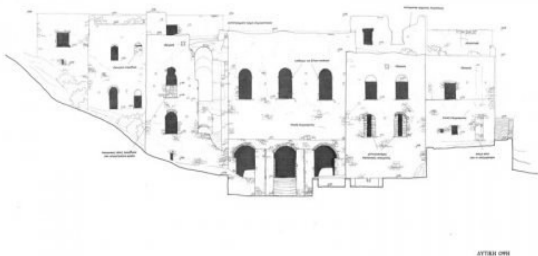
Εικ.31) Δυτική όψη εξοχικής έπαυλης Ιησουιτών στα Καλαμίτσια της Νάξου πηγή internet www.monumenta.org
