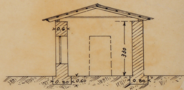
ΤΟΜΗ (α - α)
