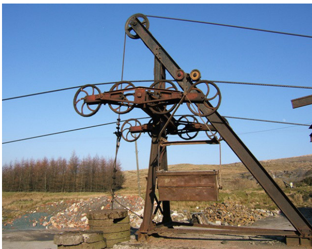
Εικ.177) μηχανήμα εναέριου σιδηρόδρομου
