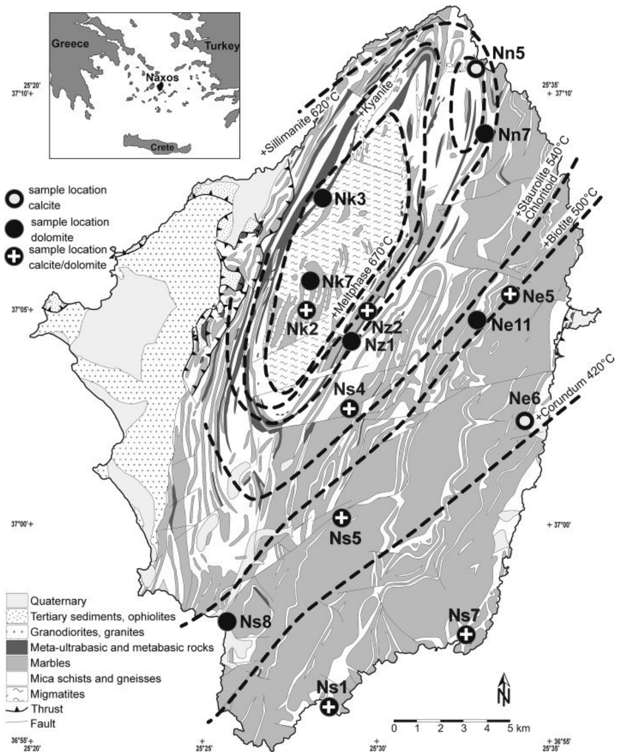
Εικ.97) Απλοποιημένος γεωλογικός χάρτης της Νάξου απο τους Jansen και Shuiling 1976.
