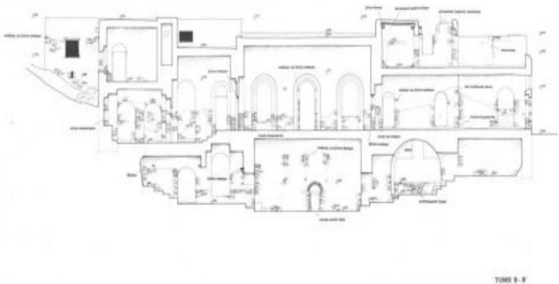
Εικ.42) Τομή β-β' εξοχικής έπαυλης των Ιησουιτών στα Καλαμίτσια της Νάξου www.monumenta.org
