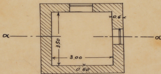
ΚΑΤΟΨΙΣ
