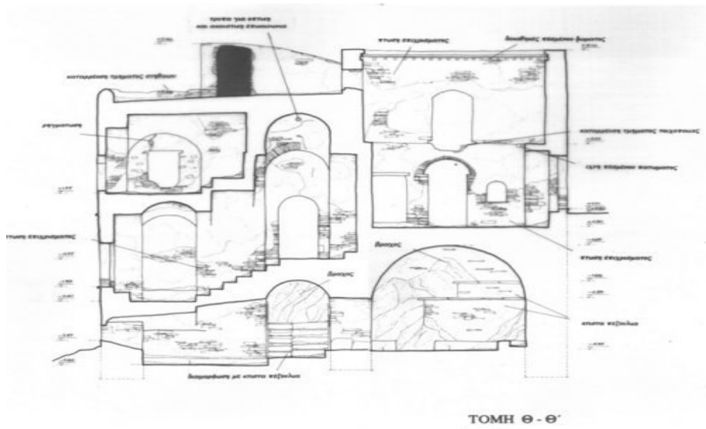
Εικ.41) Τομή α-α' εξοχικής έπαυλης των Ιησουιτών στα Καλαμίτσια της Νάξου www.monumenta.org
