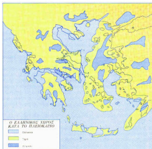
Εικ.95) ο Ελληνικός χώρος κατά το Πλειόκαινο.
