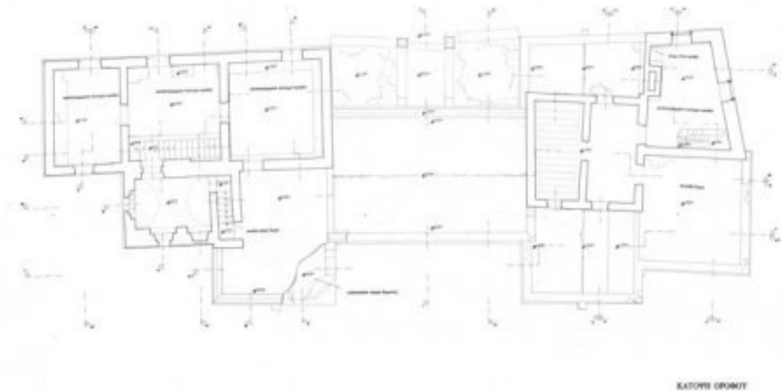
Εικ.40) Κάτοψη ορόφου εξοχικής έπαυλης των Ιησουιτών στα Καλαμίτσια της Νάξου www.monumenta.org
