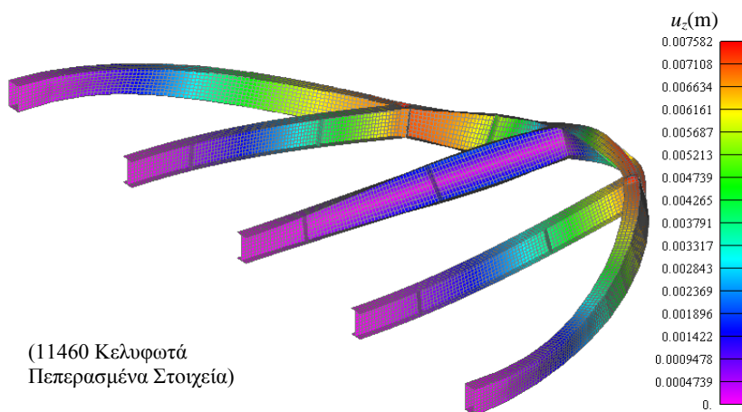
Σχ.4. Ελαστικές επιφάνειες εξεταζόμενου μεταλλικού φορέα.
