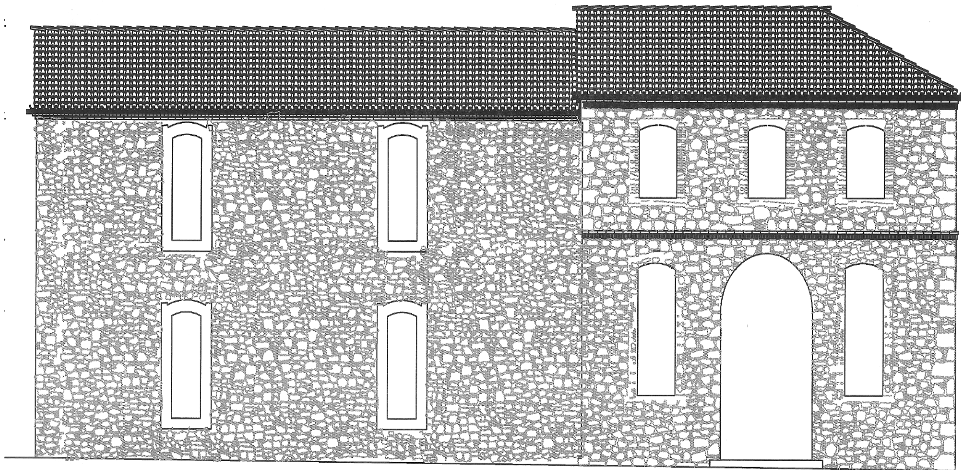
Σχ. 7. ΥΦΙΣΤΑΜΕΝΗ ΒΟΡΙΑ ΟΨΗ Πηγή: Προσωπική αποτύπωση
