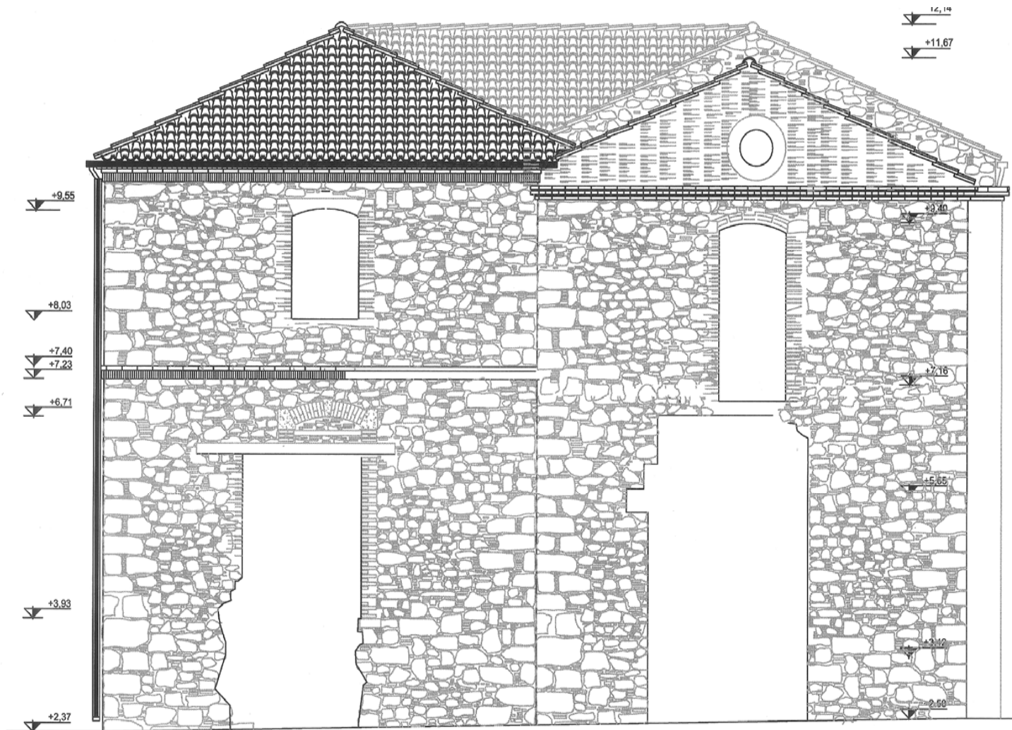
Σχ. 8. ΥΦΙΣΤΑΜΕΝΗ ΑΝΑΤΟΛΙΚΗ ΟΨΗ Πηγή: Προσωπική αποτύπωση
