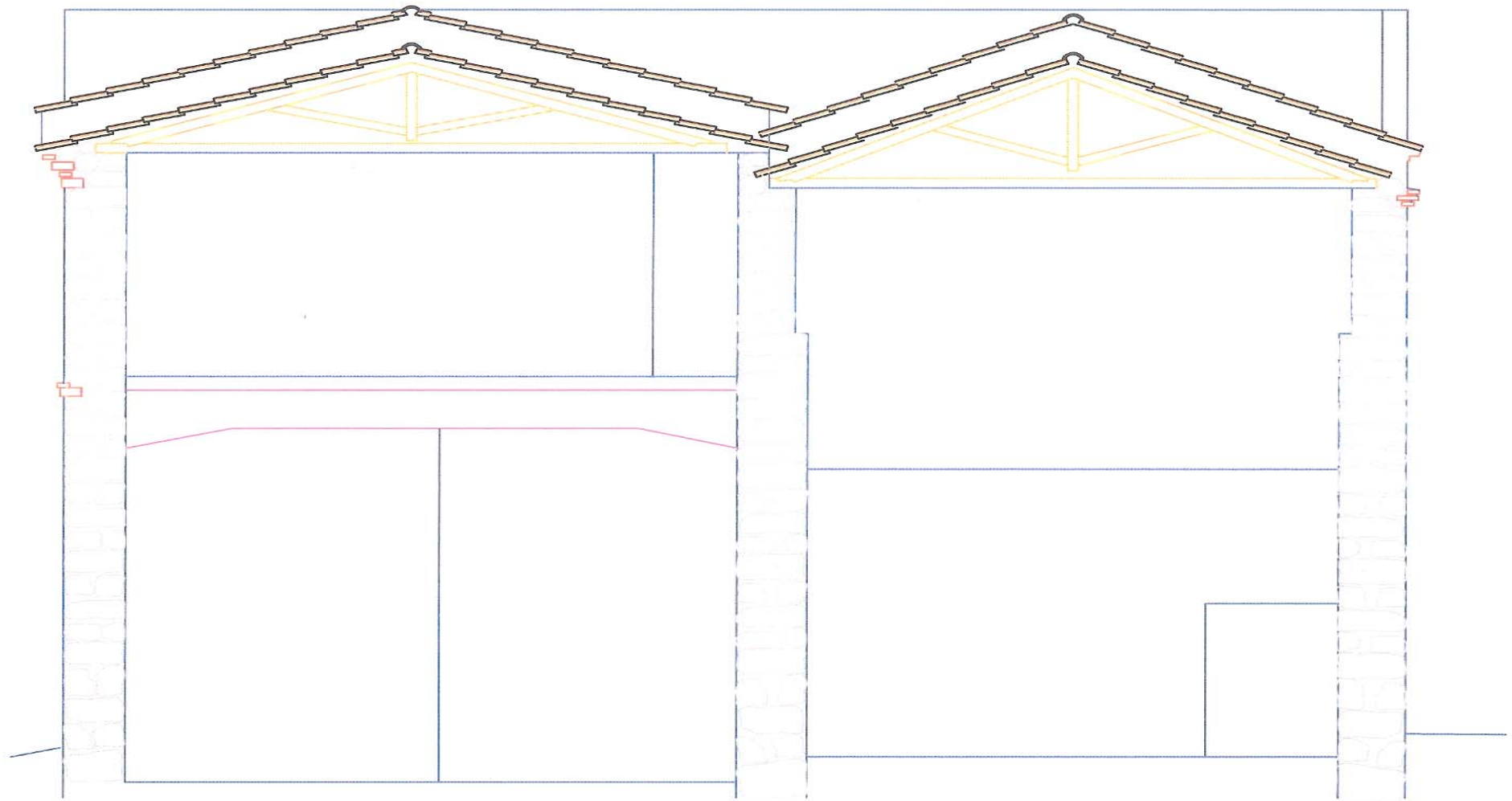
Σχ. 3, ΤΟΜΗ Α - Α Πηγή: Προσωπική αποτύπωση
