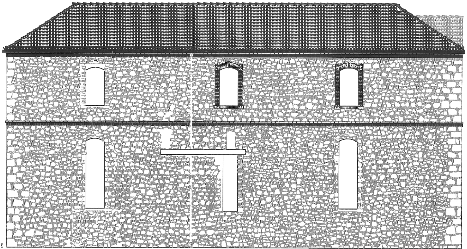
Σχ. 6. ΥΦΙΣΤΑΜΕΝΗ ΝΟΤΙΑ ΟΨΗ Πηγή: Προσωπική αποτύπωση
