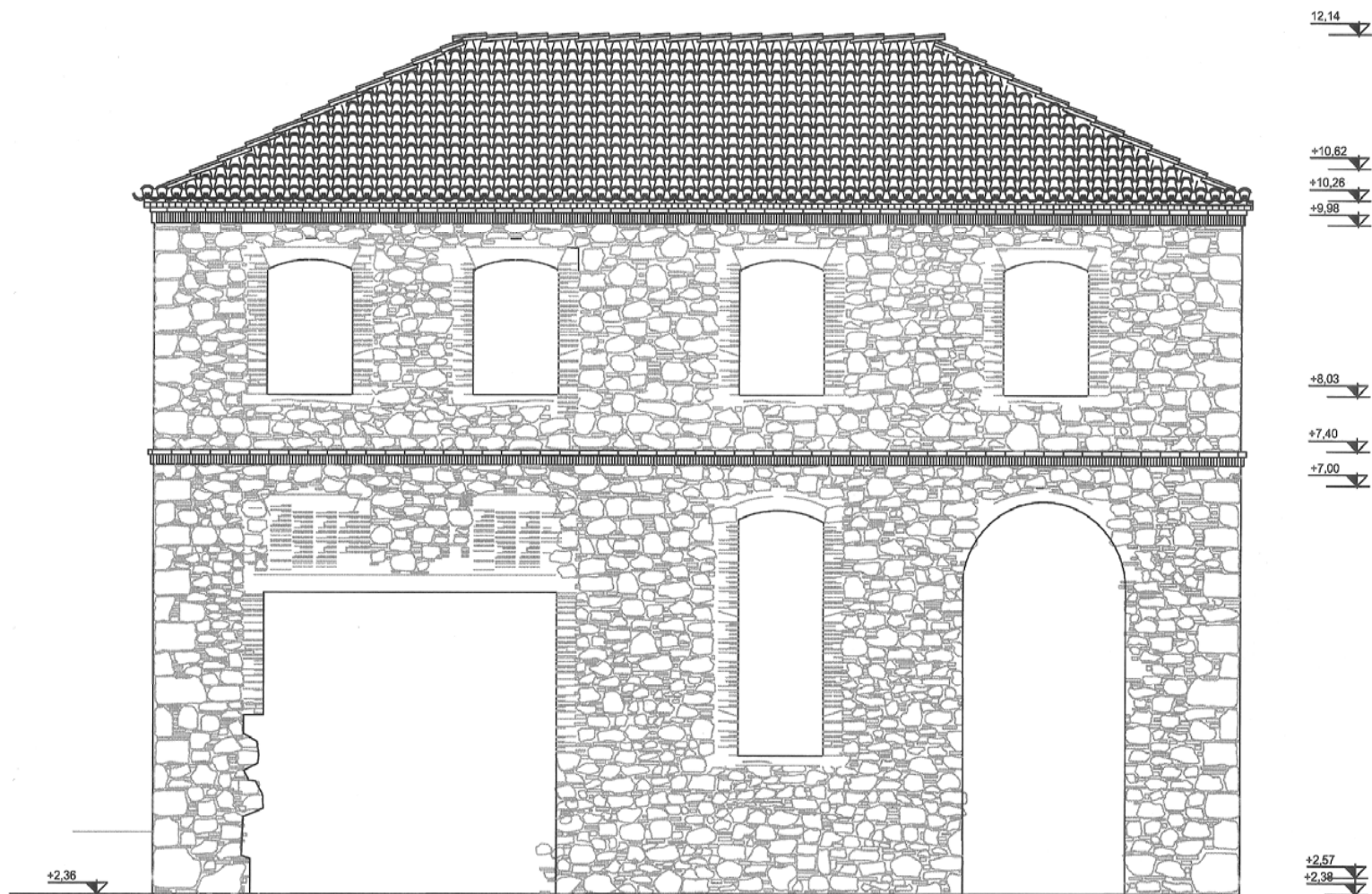
Σχ. 5. ΥΦΙΣΤΑΜΕΝΗ ΔΥΤΙΚΗ ΟΨΗ Πηγή: Προσωπική αποτύπωση
