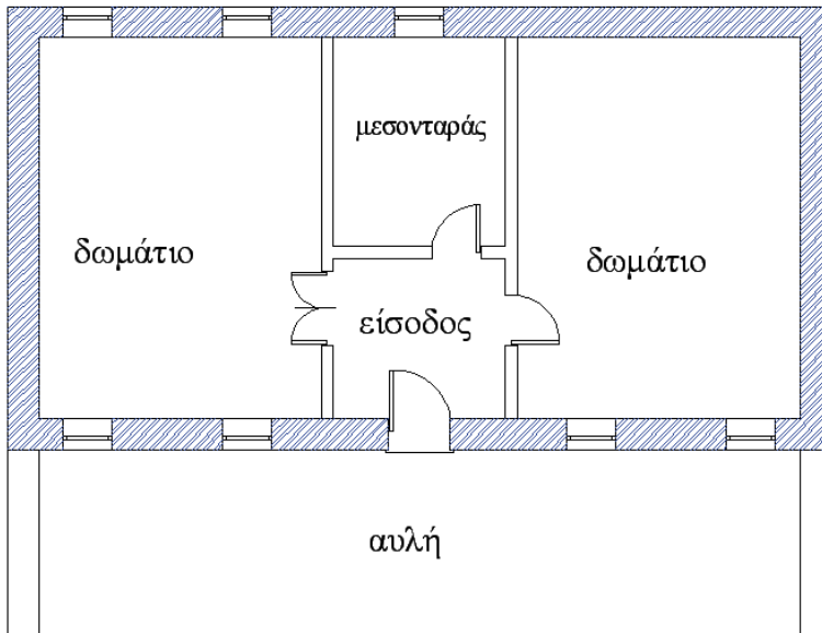
Τύπος Β ισόγειος: Κάτοψη με είσοδο, βοηθητικό χώρο και δύο δωμάτια συμμετρικά.
