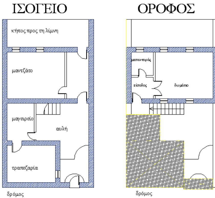
Τύπος Γ διώροφος: Δύο κατοικίες ανεξαρτητές
