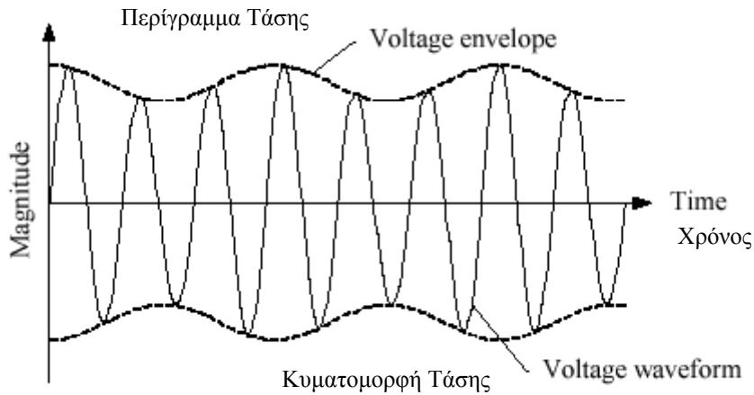
Σχήμα 3.13 Χαρακτηριστικά κυματομορφής flicker
