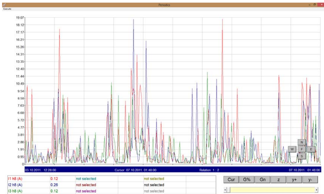
Σχήμα 3.35 8 η αρμονική για τις 3 φάσεις
