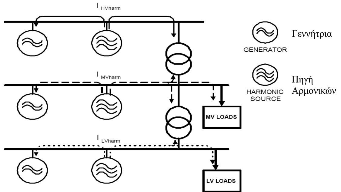
Σχήμα 3.22 Γραφική αναπαράσταση επιρροής αρμονικών που δημιουργούνται από μια πηγή αρμονικών στους υπόλοιπους καταναλωτές που είναι συνδεδεμένοι στο σύστημα ηλεκτρικής ενέργειας.
