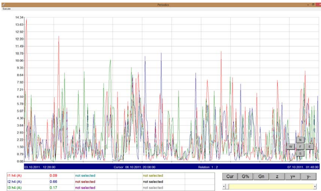
Σχήμα 3.31 4 η αρμονική για τις 3 φάσεις
