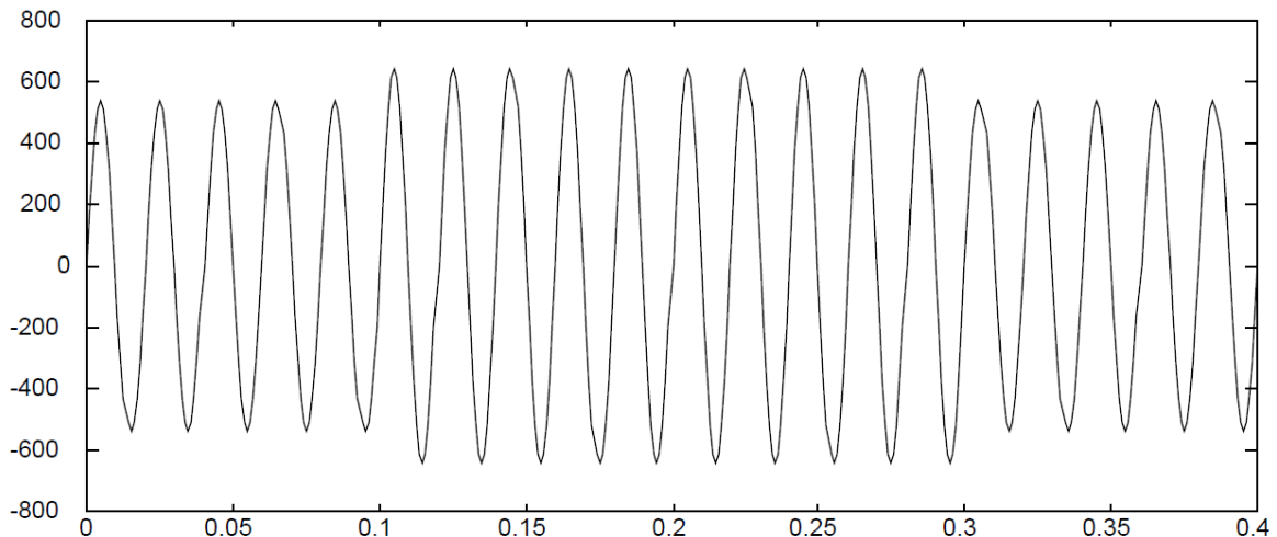
Σχήμα 3.10 Γραφική αναπαράσταση παροδικής υπέρτασης (swells)
