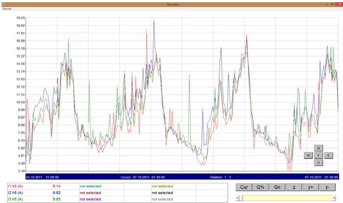
Σχήμα 3.32 5 η αρμονική για τις 3 φάσεις
