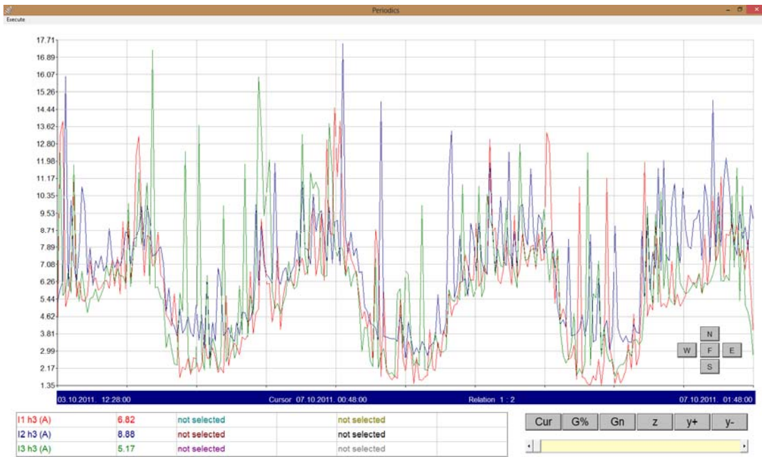
Σχήμα 3.30 3 η αρμονική για τις 3 φάσεις
