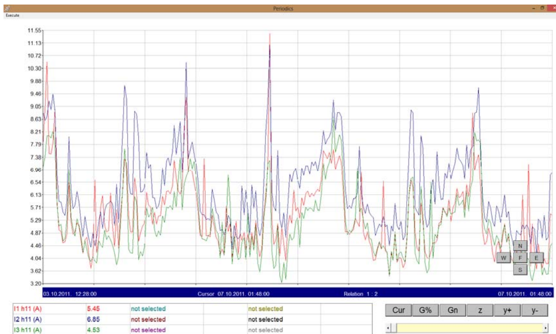
Σχήμα 3.38 11 η αρμονική για τις 3 φάσεις
