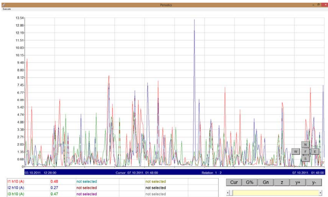
Σχήμα 3.37 10 η αρμονική για τις 3 φάσεις
