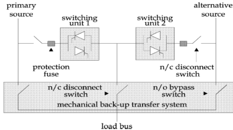
Σχήμα 3.7 Δομή του STS σε μία φάση
