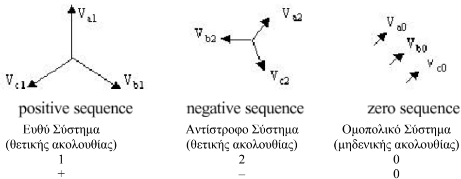
Σχήμα 3.17 Συμμετρικά στοιχεία ενός ασύμμετρου συστήματος τάσεων
