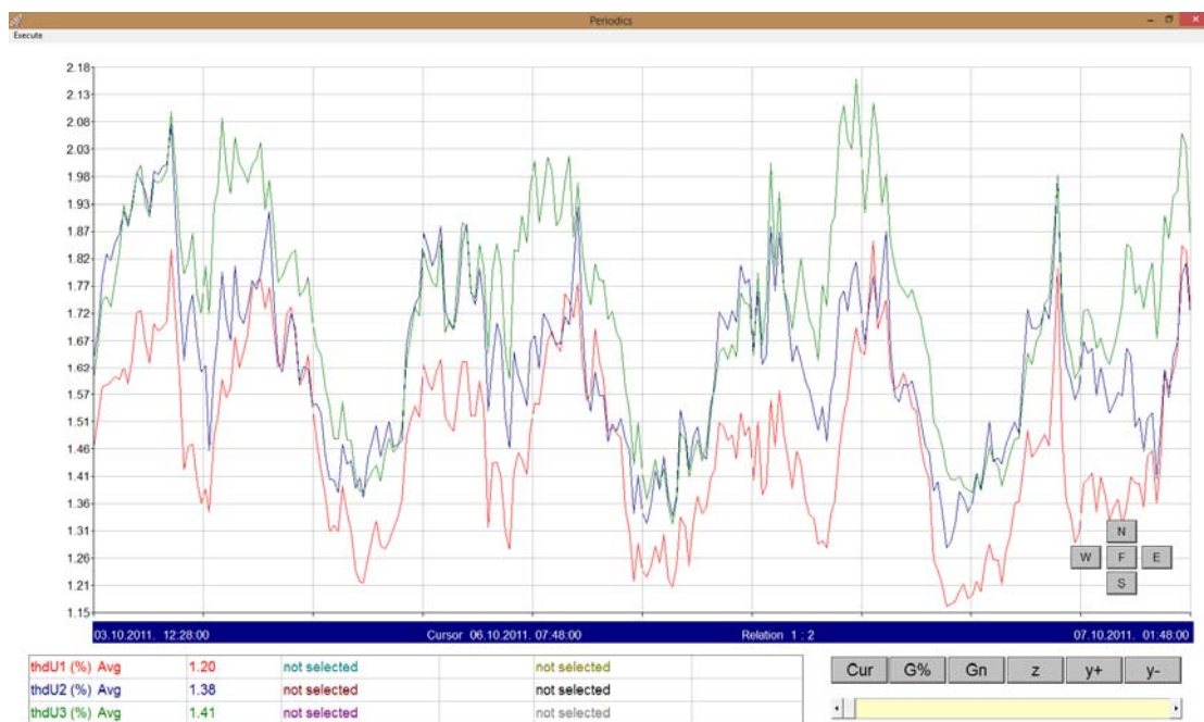
Σχήμα 3.39 Υπολογισμός του THD για τις 3 τάσεις
