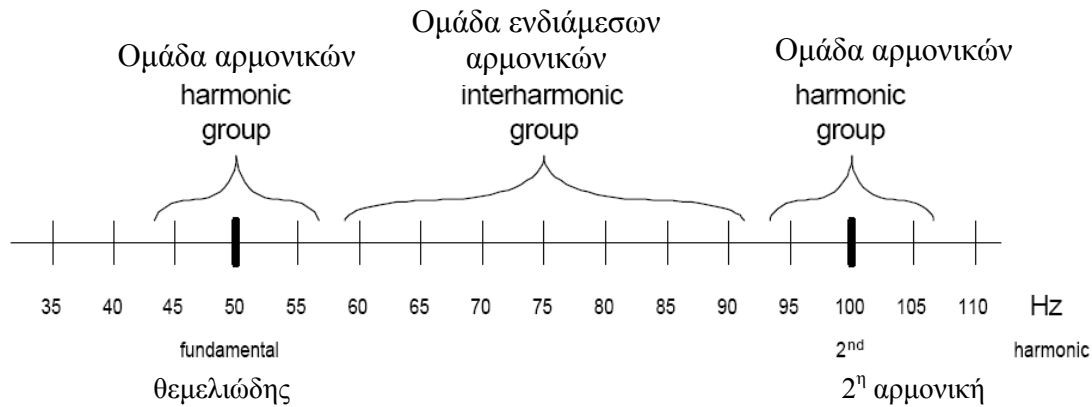
Σχήμα 3.24 Ενδιάμεσες αρμονικές στο φάσμα συχνοτήτων για DFT
