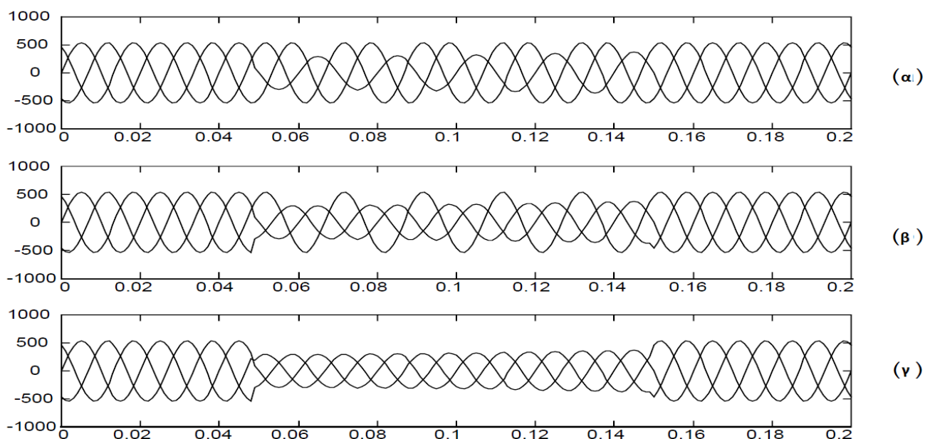
Σχήμα 3.5 Σύστημα Βυθίσεων για διαφορετικές φάσεις
