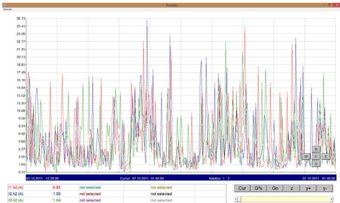
Σχήμα 3.29 2 η αρμονική για τις 3 φάσεις
