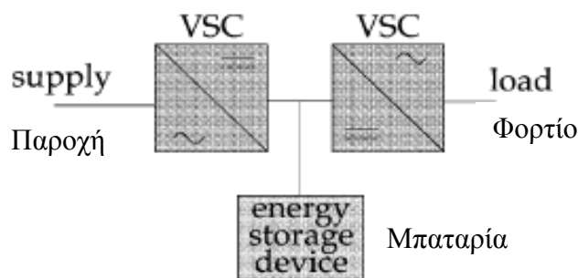
Σχήμα 3.9 Συσκευή αδιάλειπτης παροχής
