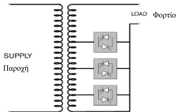
Σχήμα 3.8 SVR (Στατός Ρυθμιστής Τάσης)
