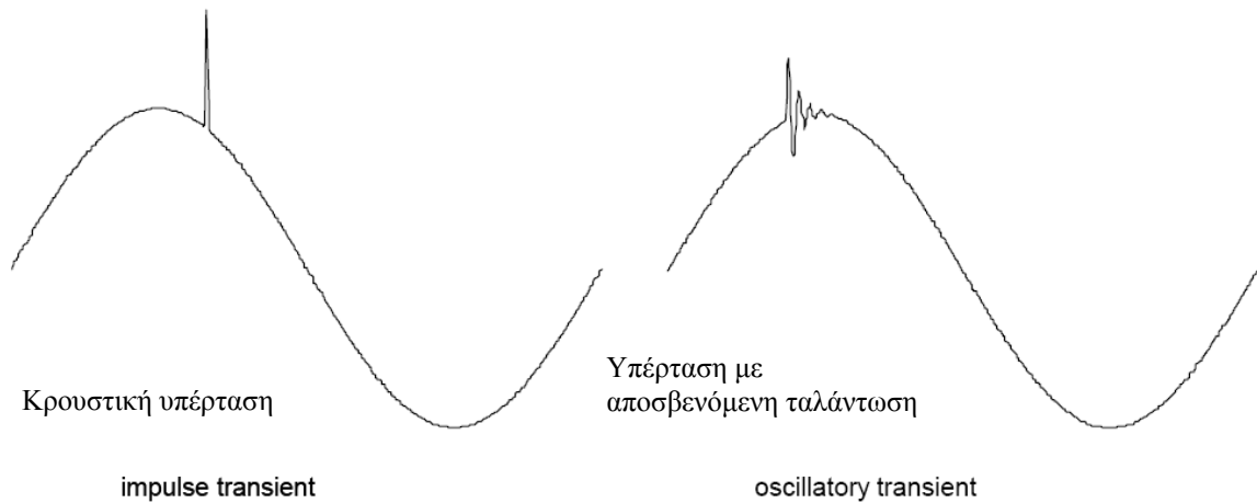
Σχήμα 3.17 Μεταγωγικές υπερτάσεις παλμικού και κλιμακούμενου τύπου
