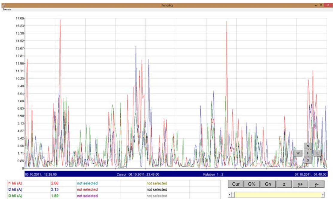
Σχήμα 3.33 6 η αρμονική για τις 3 φάσεις
