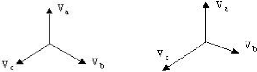
Σχήμα 3.16 Αντιπαραβολή συμμετρικού με ασύμμετρο τριφασικό σύστημα
