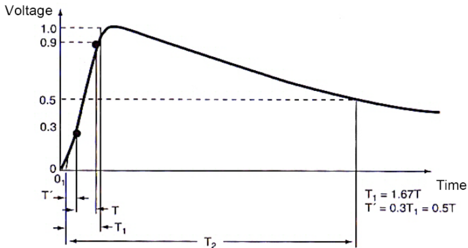
Σχήμα 3.18 Χαρακτηριστικά παλμικής διαταραχής
