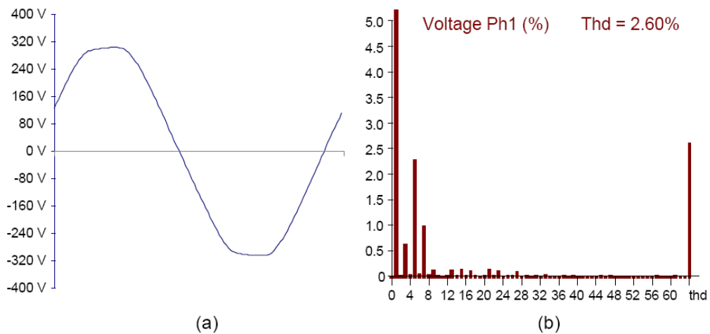
Σχήμα 3.19 Φασματική απεικόνιση μιας συνήθους κυματομορφής, αποκαλούμενης και ως πριονισμένης κορυφής
