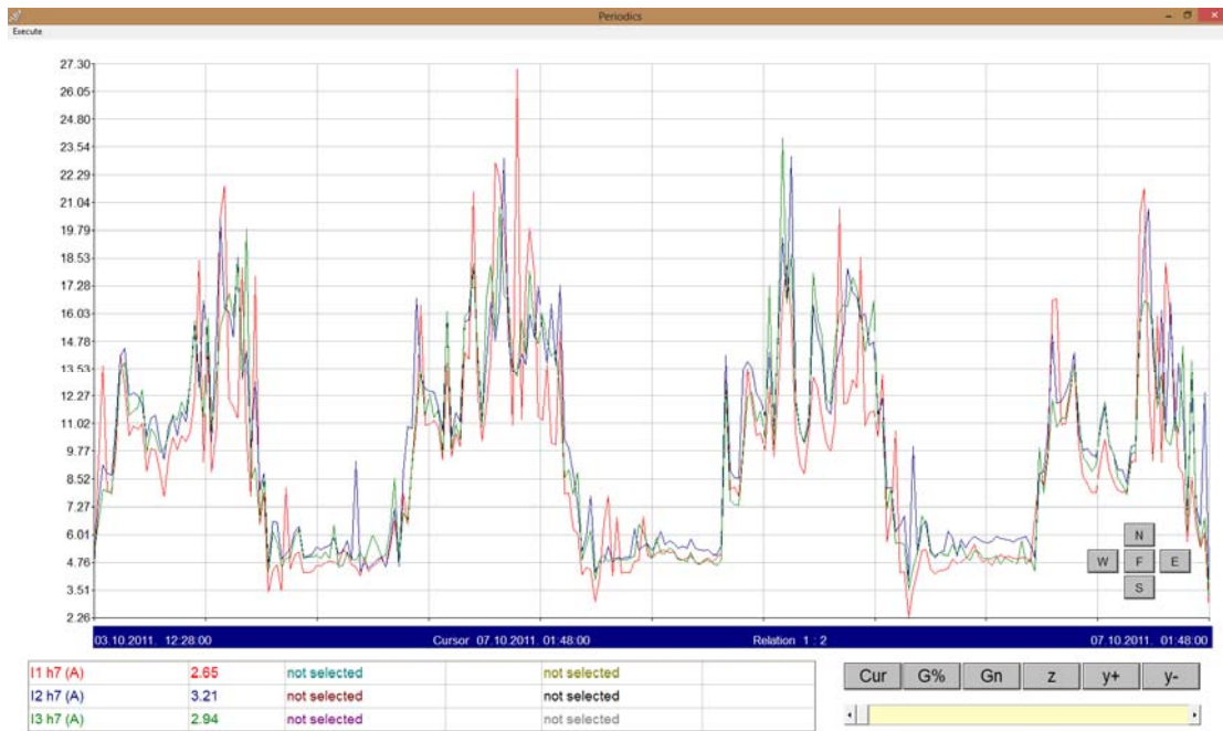
Σχήμα 3.34 7 η αρμονική για τις 3 φάσεις
