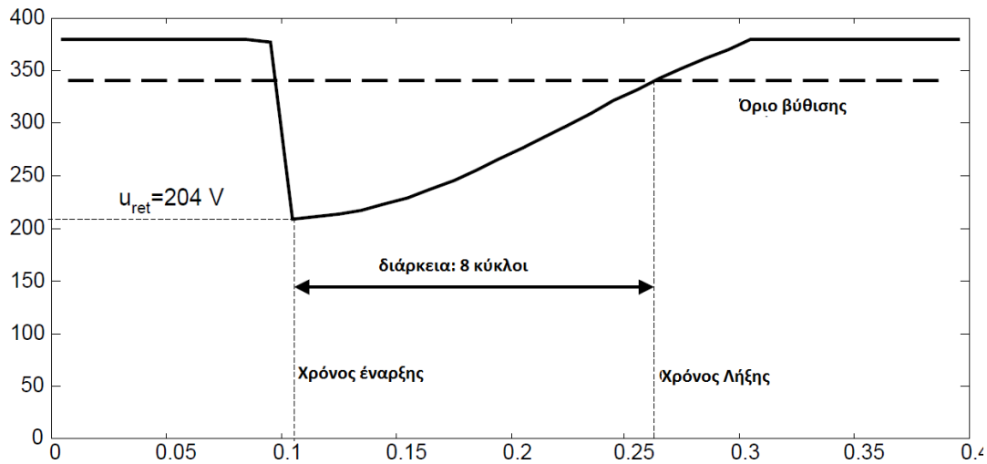
Σχήμα 3.4 Χαρακτηριστικά Βύθισης Τάσης
