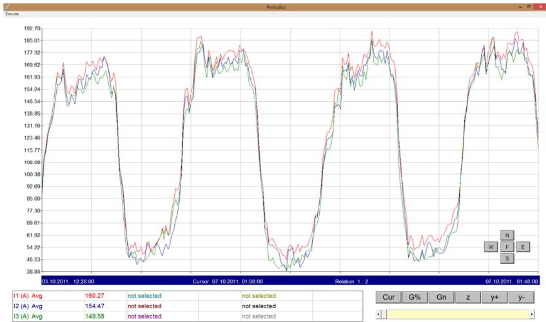
Σχήμα 3.28 Συγκριτικό διάγραμμα με τις μέσες τιμές των ρευμάτων (με κόκκινο η μέση τιμή του ρεύματος I1, με πράσινο η μέση τιμή του ρεύματος I3 και με μπλε η μέση τιμή του ρεύματος I2)
