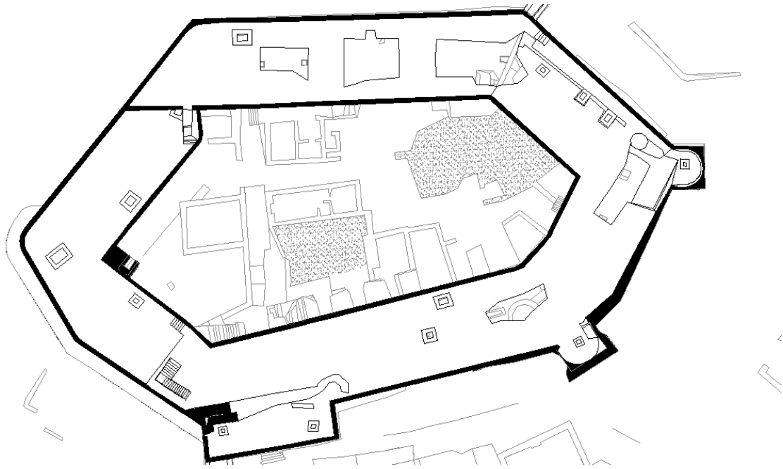
Εικόνα 25 Το Κάστρο περιβάλλεται από δύο περιβόλους. Ο εξωτερικός έχει σχήμα πολυγωνικό, ενώ ο εσωτερικός έχει σχήμα ακανόνιστου εξαγώνου.
